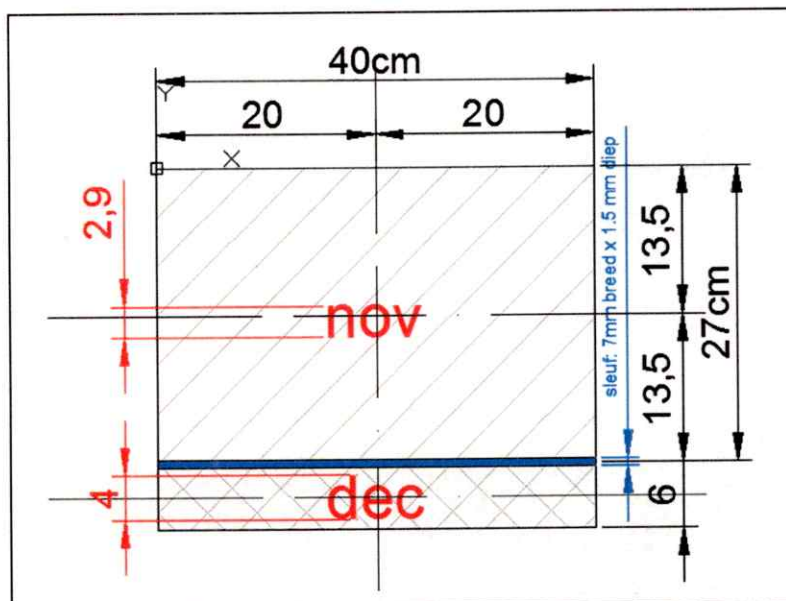
Fig. 3. Detailtekening van de maandnamen november/december op de datumlijn.
