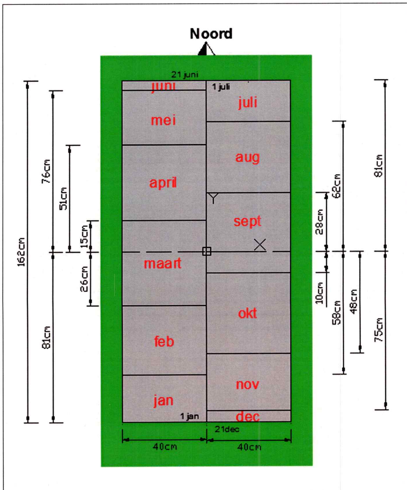
Fig. 2. Grondplan van de datumlijn.
