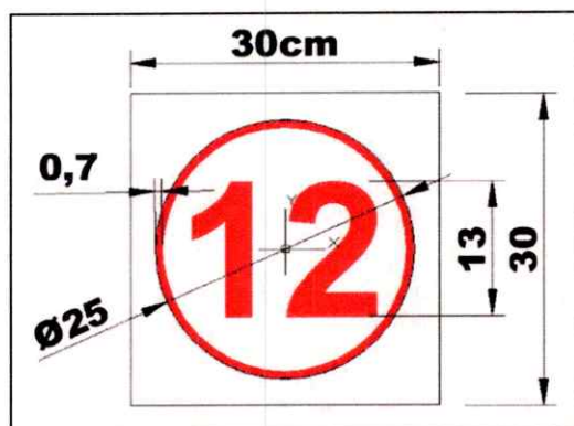
Fig. 4. Detailtekening van de 12 uur-tegel.
