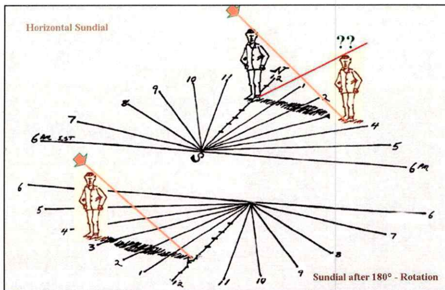
Fig. 10. Zonnewijzerconstructie geroteerd over 180^\circ . (J.U. Bel - gemodificeerd)
